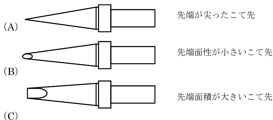
図 1. 各種こて先
